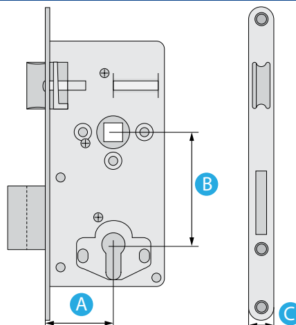
- brava GE-GE 8 cm.sa podizačem
